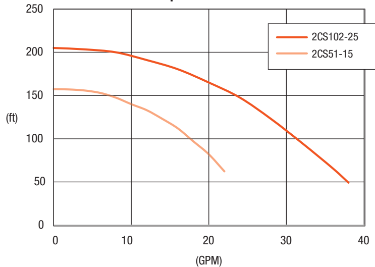
Curva de Operación de las bombas
