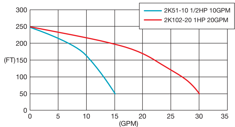
Curva de Operación de las bombas (Rango 30-100 PSI)
