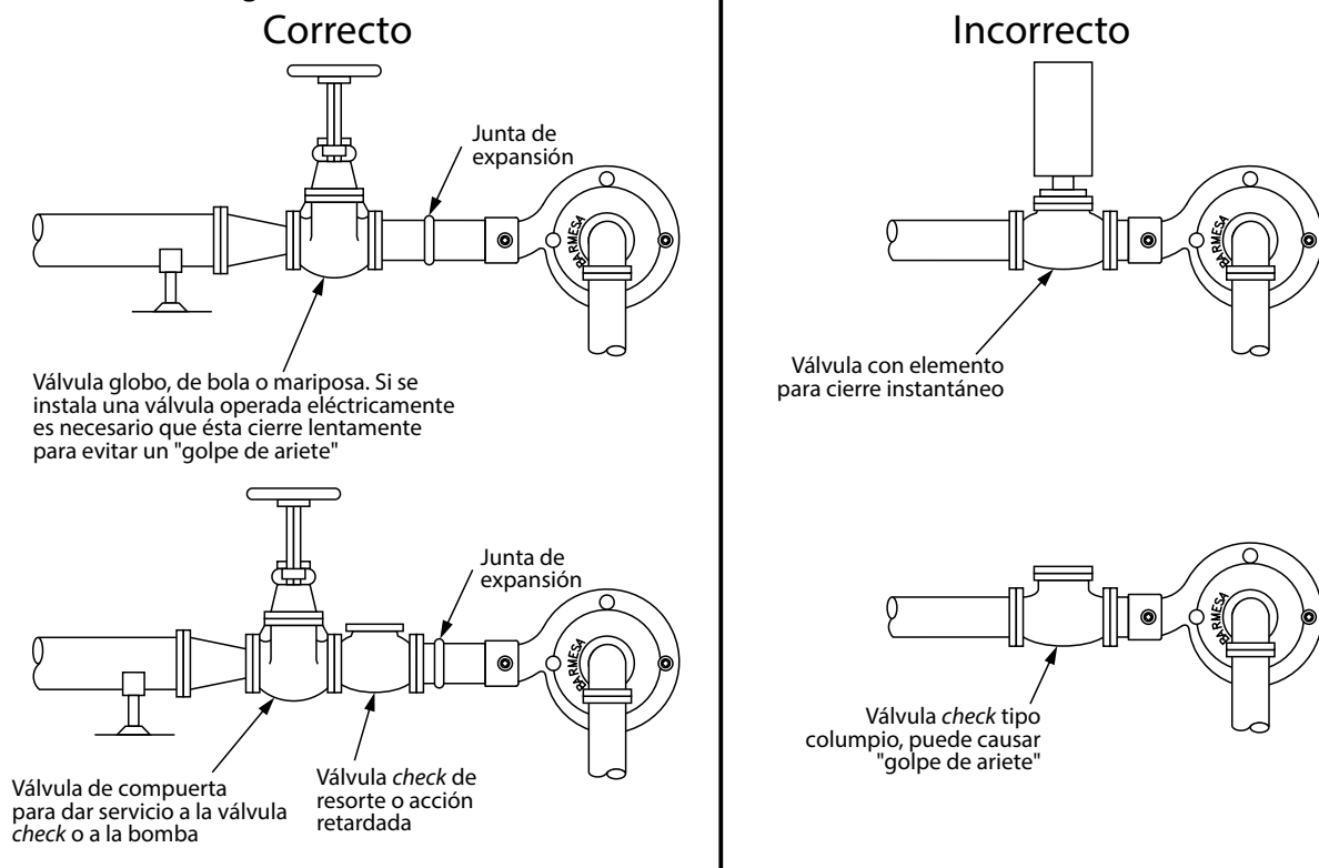
Figura 6 Tubería de descarga
